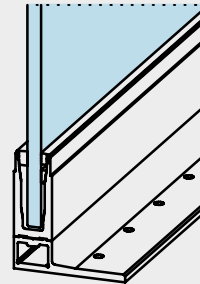
Profilo di base con sostegno rialzato a piede largo Standard Profile with height and base spacer, fitted one side only Základní profil s vestavbou s širokou patkou pro nástavbu podlahy
