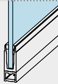
Profilo di base con sostegno rialzato Standard Profile with height spacer Základní profil s vestavbou pro nástavbu podlahy
