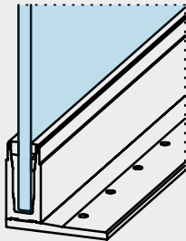
Profilo di base con sostegno rialzato per montaggio a filo muro Standard Profile with extended base leg, fitted one side only, top mounted Základní profil s vestavbou pro hranovou montáž pro nástavbu podlahy
