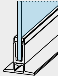
Profilo di base con sostegno per montaggio a filo muro Standard Profile with spacer plate with height and base spacer, centrally fitted
