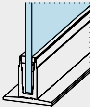
Profilo di base con sostegno a piede largo Standard Profile with spacer plate, centrally fitted
